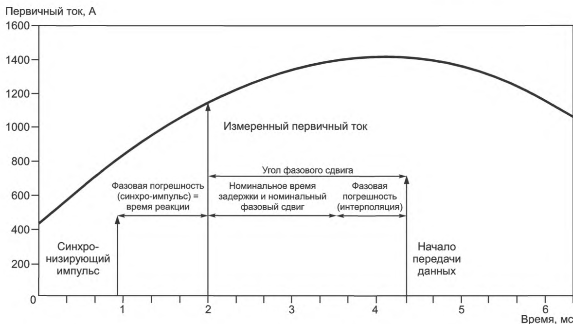
Рисунок В.4 — Определение фазовой погрешности для цифрового интерфейса
