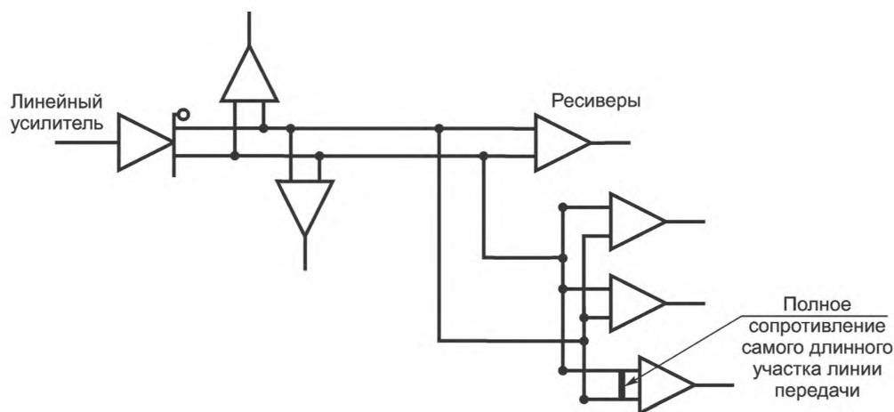
Рисунок 9 — Организация линии передачи в форме гирляндной цепи
