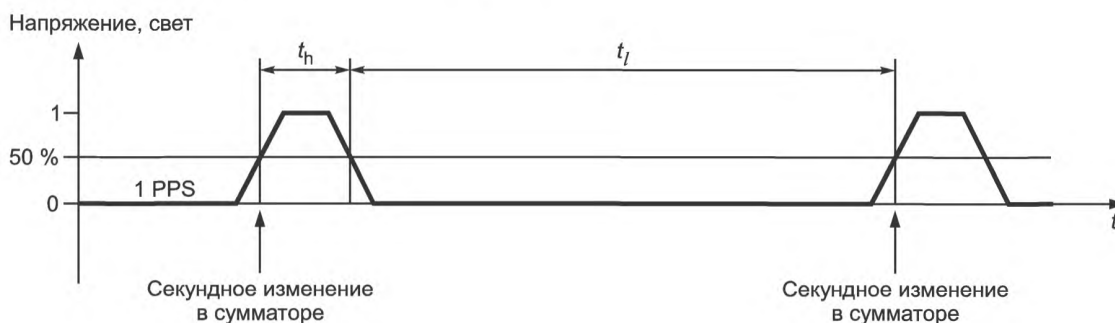
Рисунок 14 — Форма синхроимпульса
